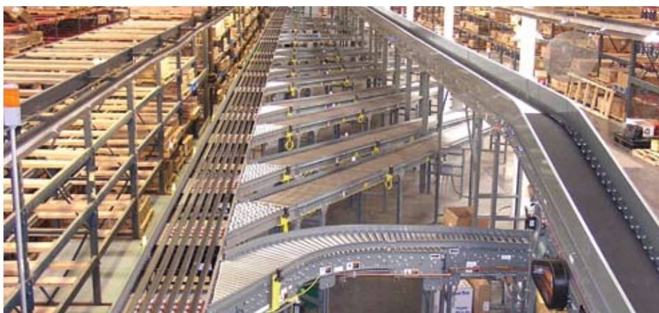
Transportadores de correia motorizados
