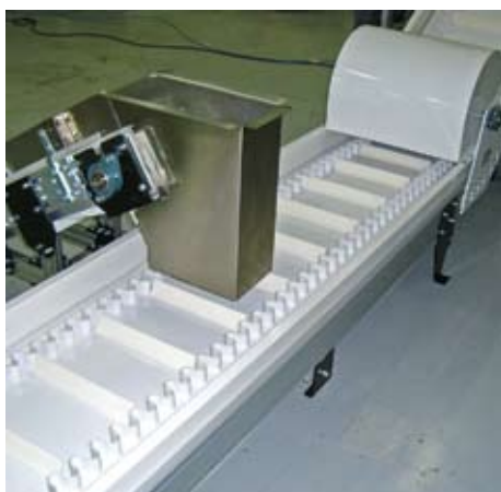
Transportador de correia sanitária
